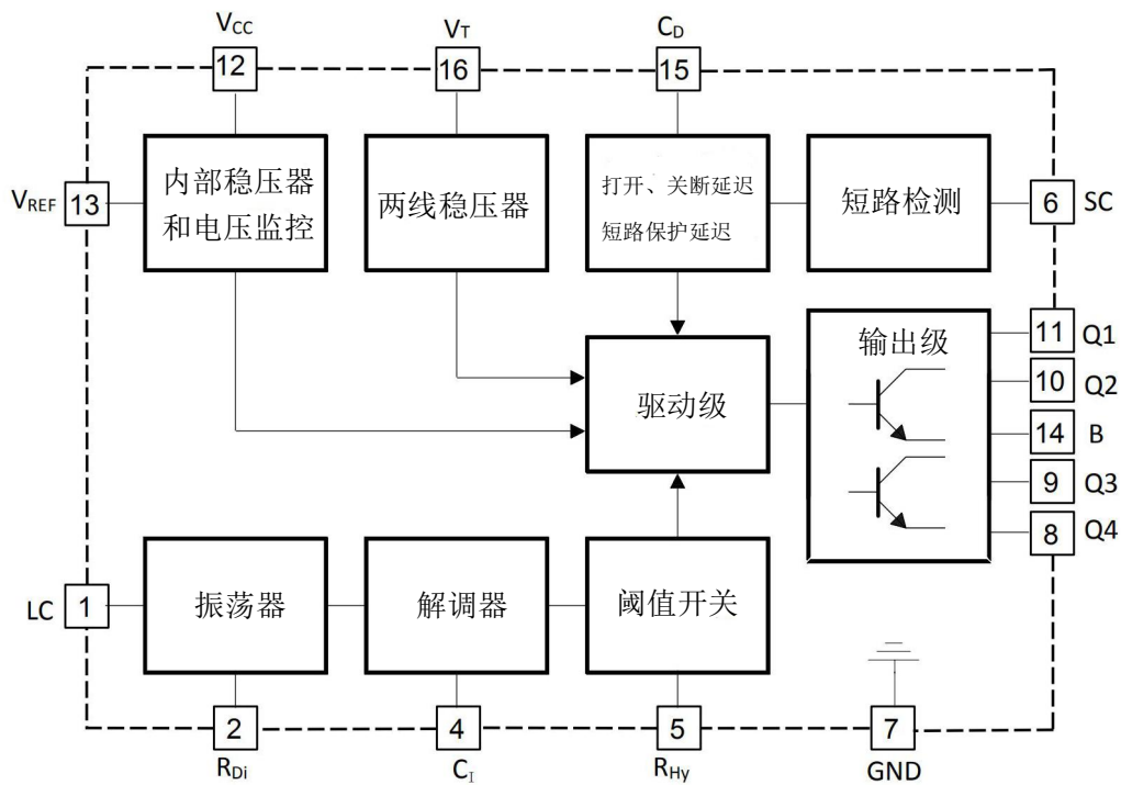
图 1. LDA505 内部结构框示意图
