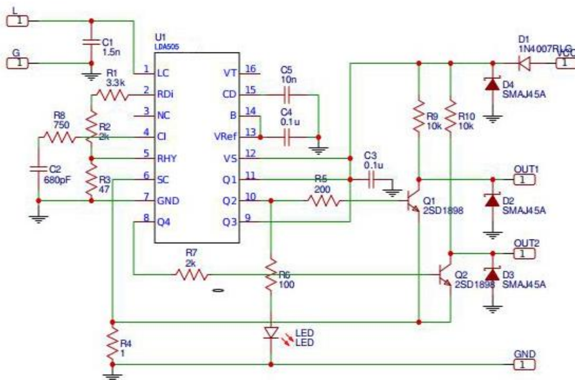
应用电路图
