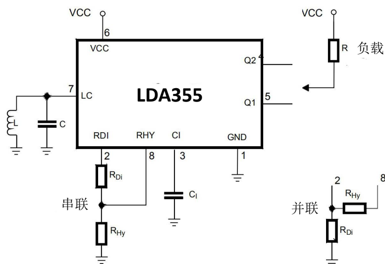
图 2. 工作原理图
